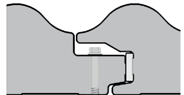
PF 600 - 60 MO Pormenor de montagem Detalle de montaje
